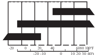
SAE VISCOSITEITSKLASSEN
