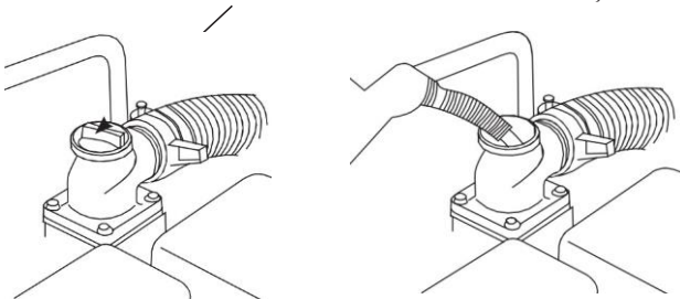
BOUCHON DE REMPLISSAGE D'EAU D'AMORÇAGE
